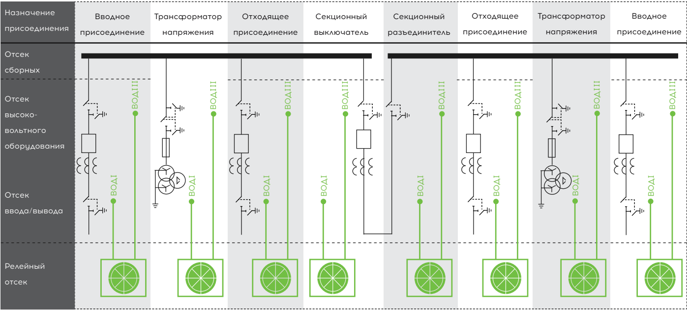
Пример размещения датчиков ВОД в ячейках КСО
