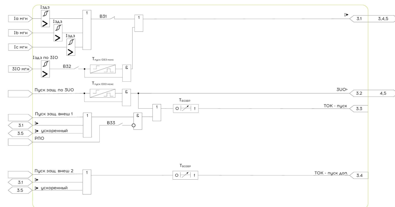
Функциональная схема алгоритма №3 «Пуск по току»
