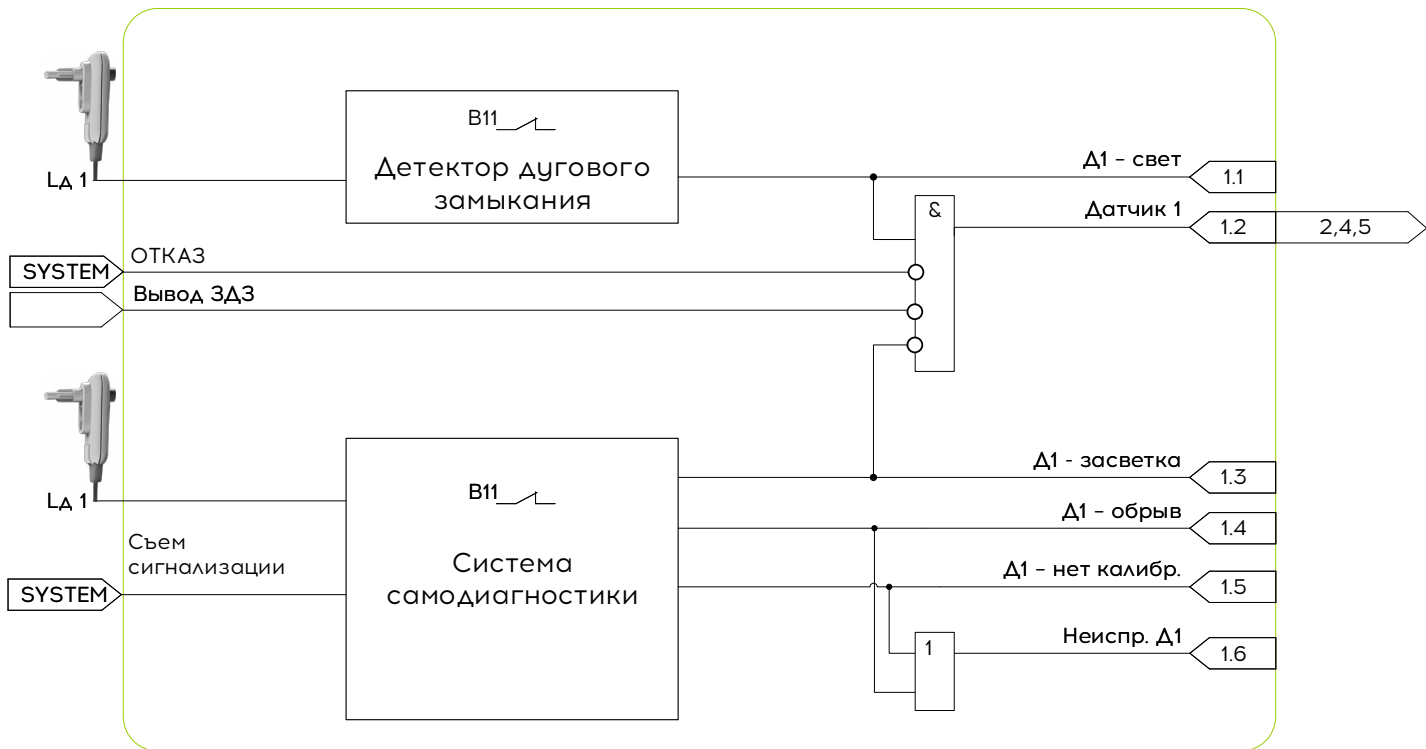
Функциональная схема алгоритма №1 «Обработка сигналов и диагностика датчиков»
