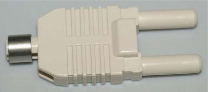
2. Соединитель с обжимным кольцом, дуплекс - 10 шт.
