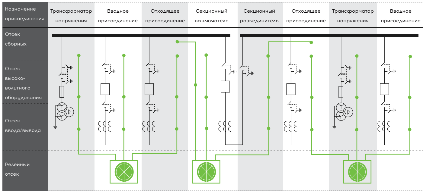
Пример размещение датчиков ТЕКИЛА в ячейках КСО
